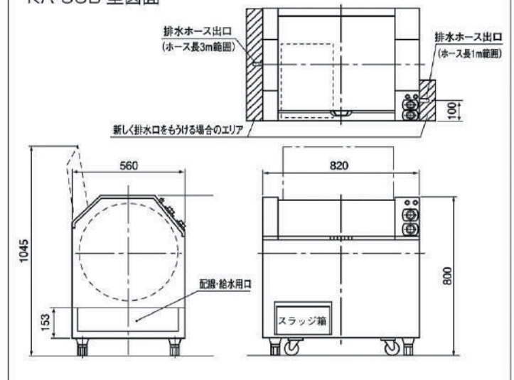
KA-60B 型図面
